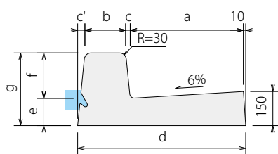
●L型街渠ブロック
