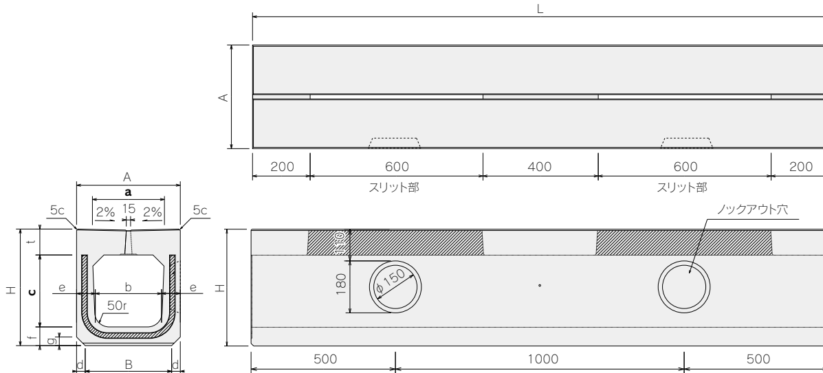
●寸法および重量表
