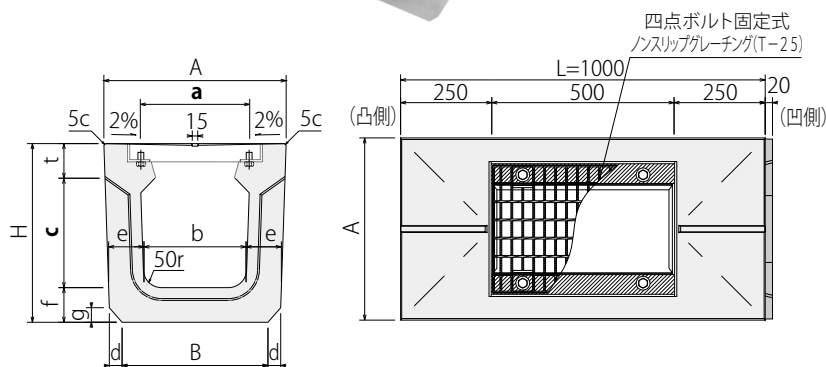
●寸法および重量表 (管理用グレーチング付)
