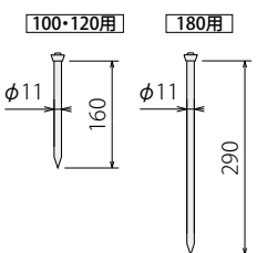
アスファルト舗装用アンカーピン
