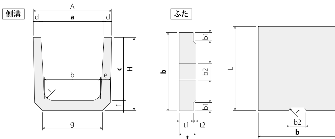
●側溝／寸法および重量表
