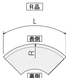
●歩車道境界ブロック 片面 R部施工 使用本数表
