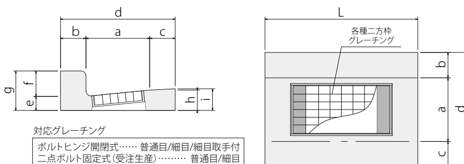
●寸法および重量表
