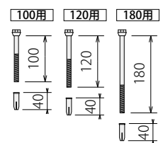
コンクリート舗装用アンカーピン
