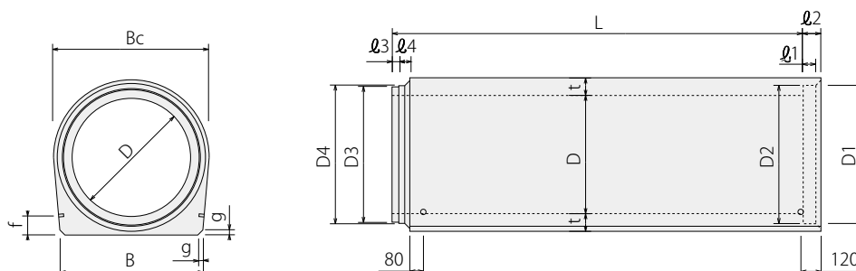
●寸法および重量表
