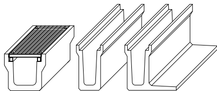
インサート付 落ちふた3種 (ボルト固定G付)
