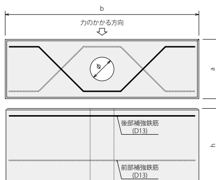
b ≥ 1.3mの場合
