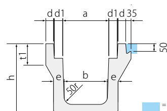
●落ちふた式 U形側溝3種
