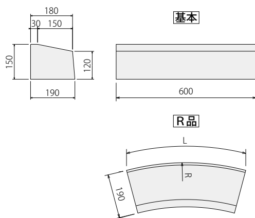
●Eブロック R部施工 使用本数表
