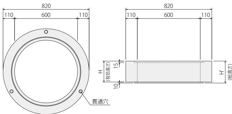
●寸法および重量表
