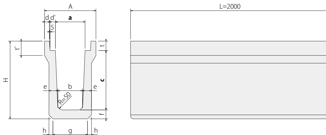
●寸法および重量表
