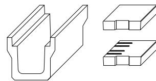
落ちふた式U形側溝 ノングレートふた
