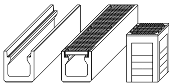
YS側溝シリーズ 標準・乗入G付・YS柵
