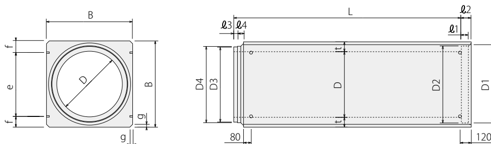
●寸法および重量表
