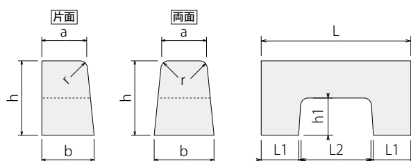
●歩車道境界ブロック（水抜き） 寸法および重量表
