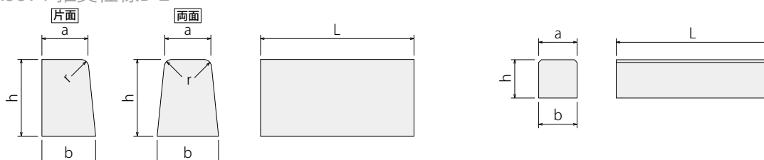
●歩車道境界ブロック・地先境界ブロック 寸法および重量表
