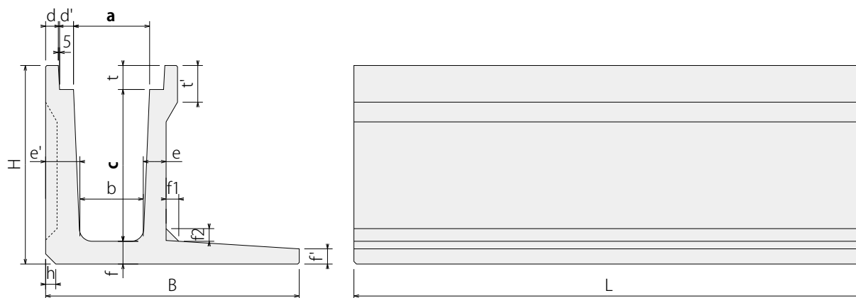
●寸法および重量表
