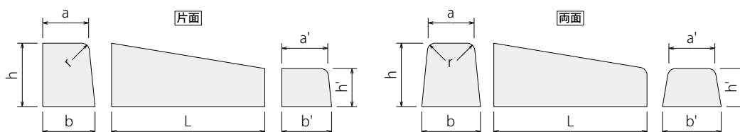
●歩車道境界ブロック（乗入れ） 寸法および重量表
