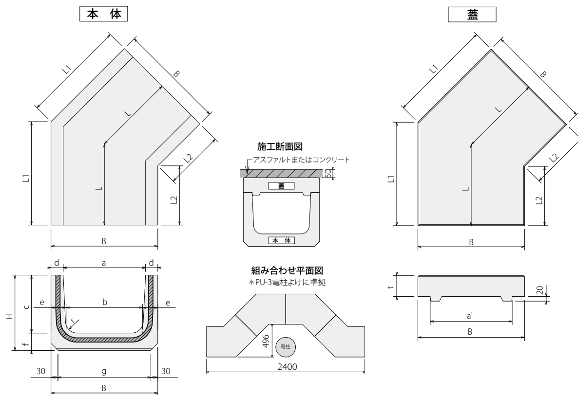
●寸法表 電柱よけコーナーおよび蓋(4分割暗渠型)
