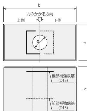
b ≤ 1.2mの場合
