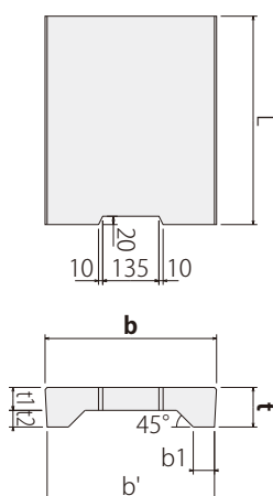
●1種 (PC3型)
