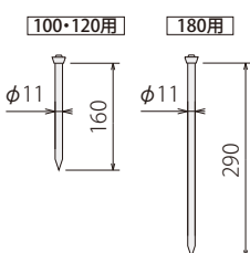
アスファルト舗装用アンカービン
