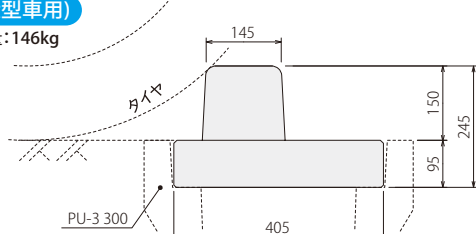
300 (大型車用)
