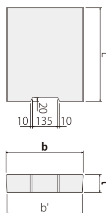
●3種 (PC4型)
