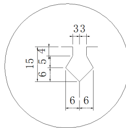
目地部詳細図
