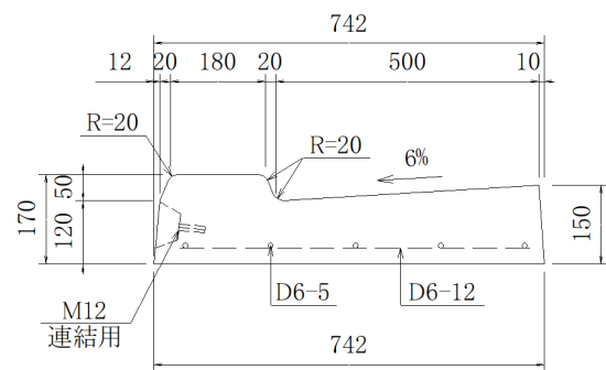
端面図(切下側)
