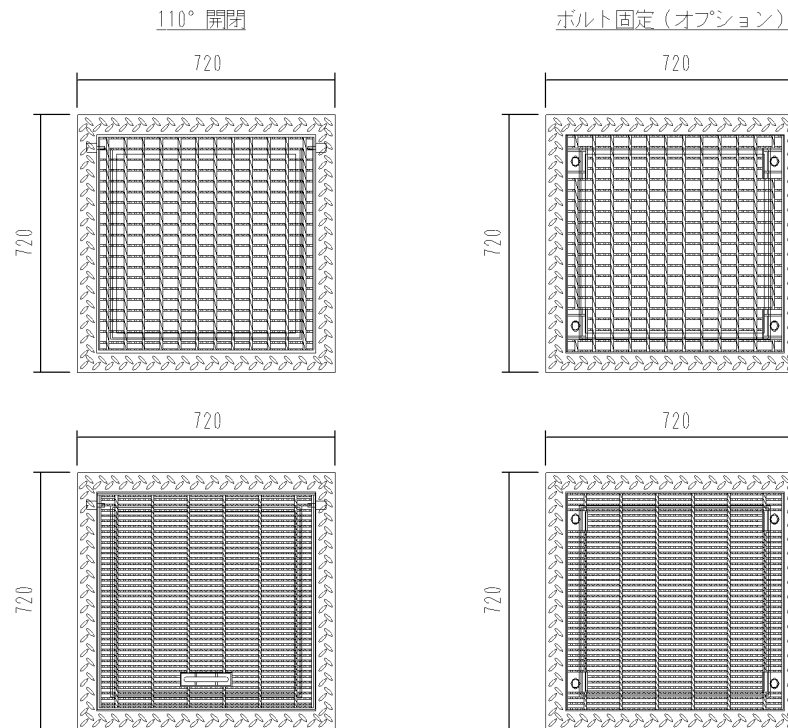
A S型 可変側溝用柵 500×500×1200 1基当たり材料表
