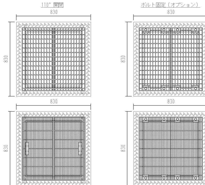
A S型 可変側溝用柵 600×600×1800 1基当たり材料表
