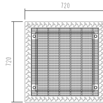
A S型 可変側溝用柵 500×500×800 1基当たり材料表
