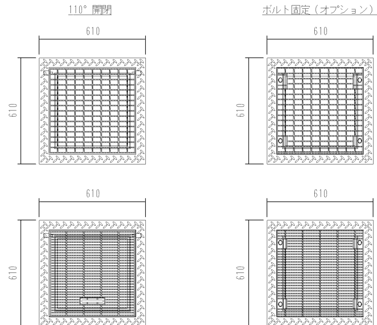
A S型 可変側溝用柵 400×400×500 1基当たり材料表
