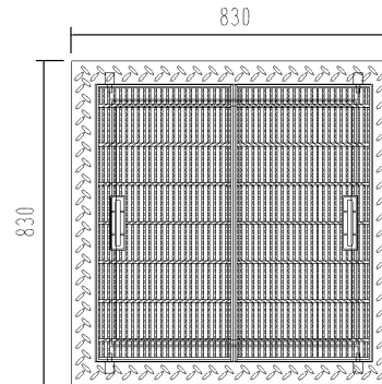
A S型 可変側溝用柵 600×600×1400
