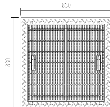
A S型 可変側溝用柵 600×600×1200
