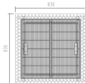
A S型 可変側溝用柵 600×600×800
