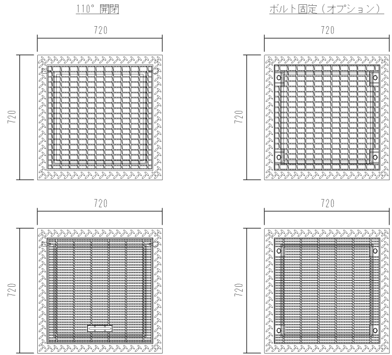
A S型 可変側溝用柵 500×500×1400 1基当たり材料表
