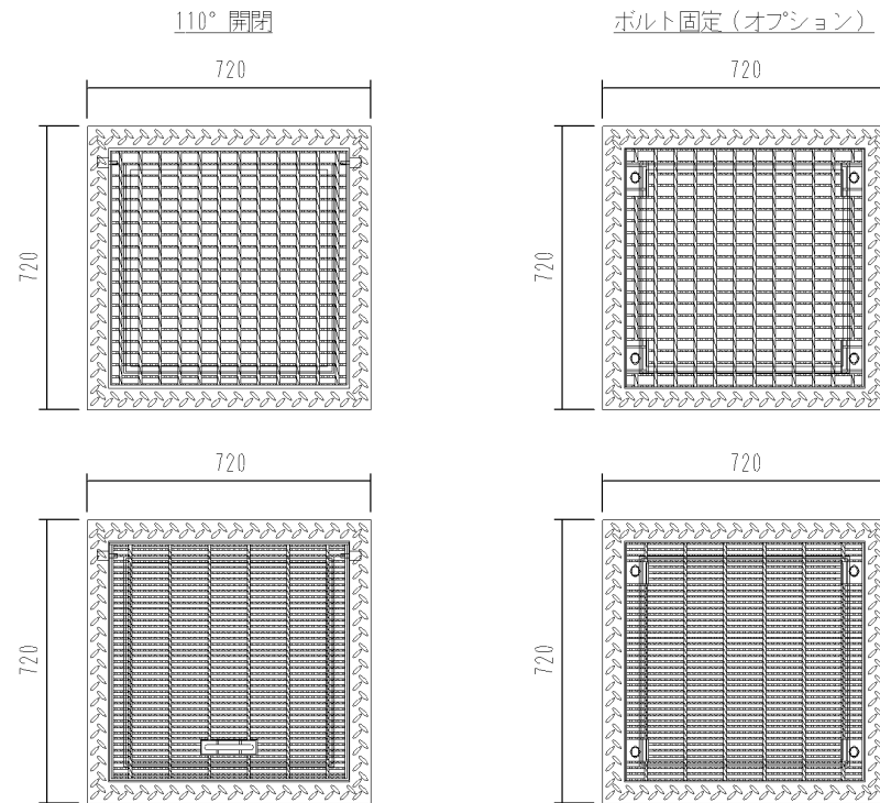
A S型 可変側溝用柵 500×500×600 1基当たり材料表
