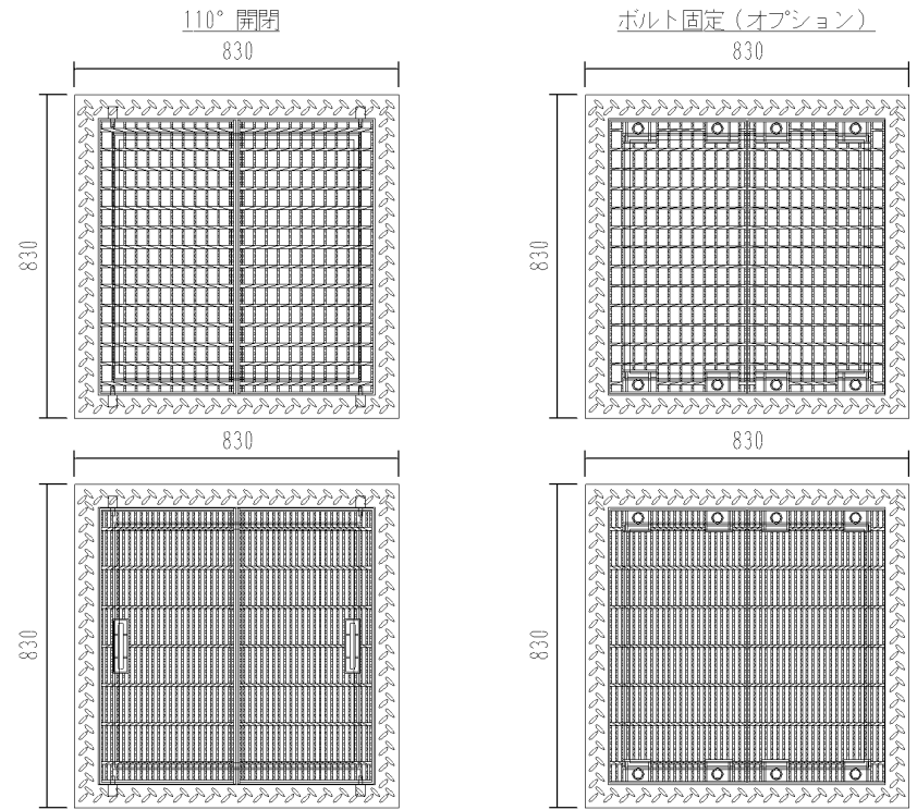
A S型 可変側溝用柵 600×600×1600 1基当たり材料表
