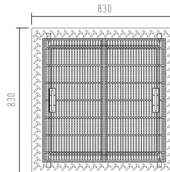
A S型 可変側溝用柵 600×600×1000 1基当たり材料表
