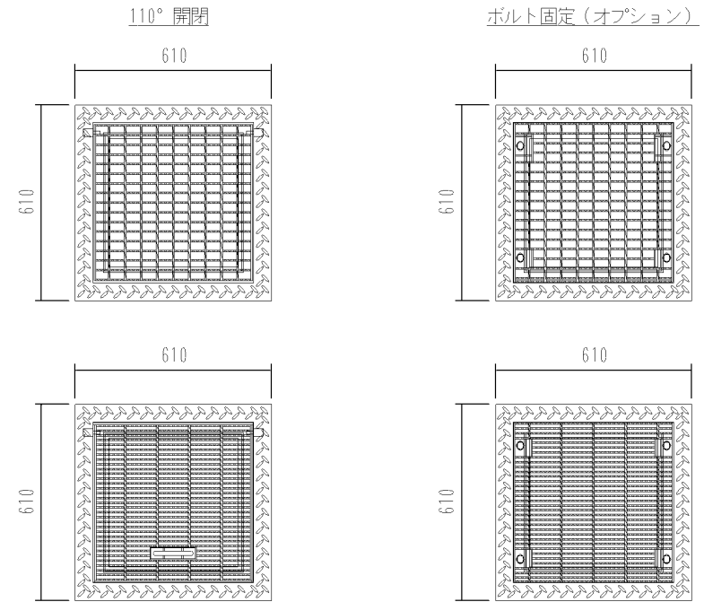
A S型 可変側溝用柵 400×400×1200 1基当たり材料表
