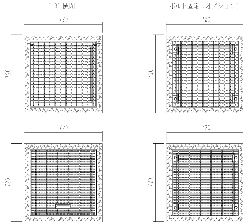
A S型 可変側溝用柵 500×500×1000 1基当たり材料表
